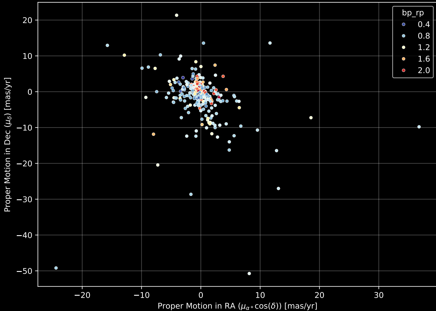
GALAH DR4 Field: [9027] Proper Motion Diagram (n= 252)
