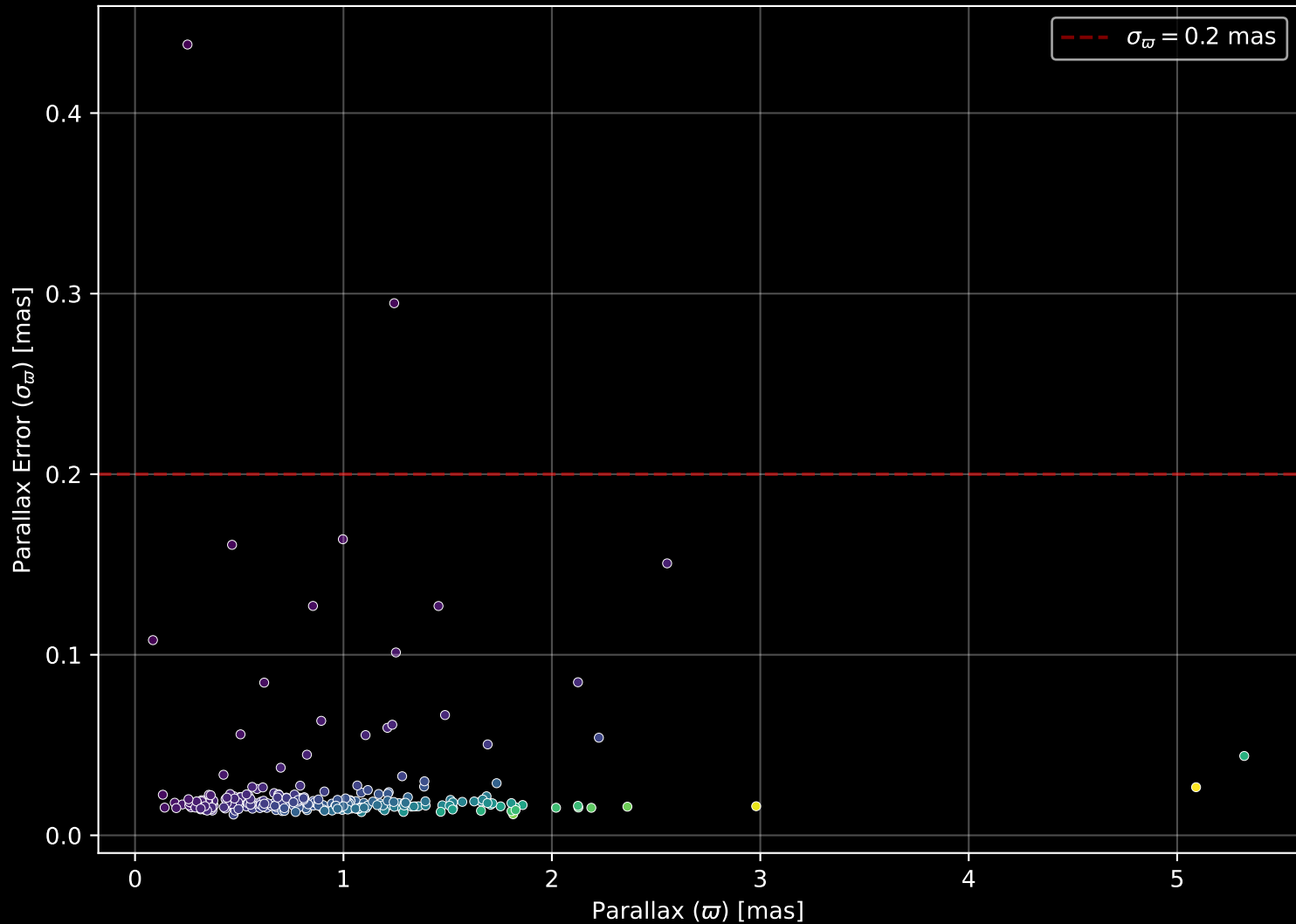
GALAH DR4 Field: [9027] Parallax Quality (n= 252)
