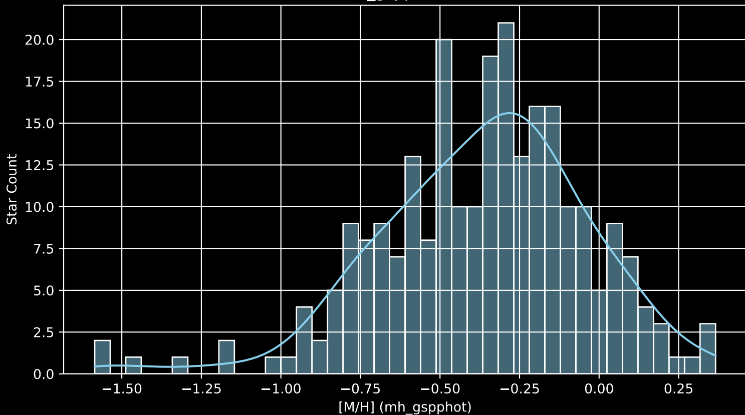
GALAH DR4 Field: [9027] [M/H] (mh_gspphot) (n= 251)
