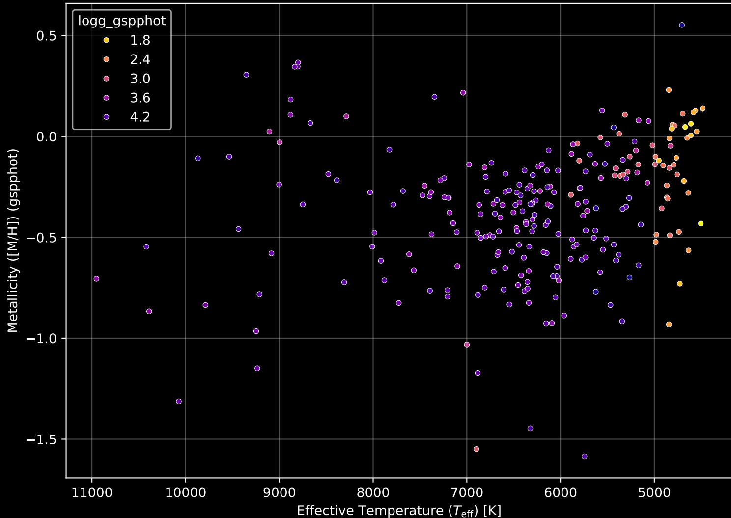
GALAH DR4 Field: [9027] Stellar Population Parameters (n= 252)
